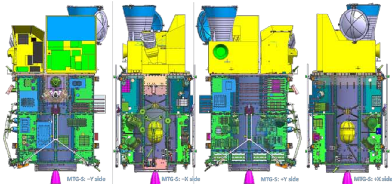
Darstellungen der Satellitenplattform (oben), des MTG-Sounder Satelliten von 4 Seiten (links) sowie der Instrumente IRS und FCI auf der folgenden Seite / Drawings of the satellite platform (above), the MTG-Sounder Satellite in a 360° view (left) and the instruments IRS and FCI on the following page.....
